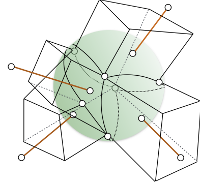
(d) The resulting scaffold mesh of Fig. 4(c)
